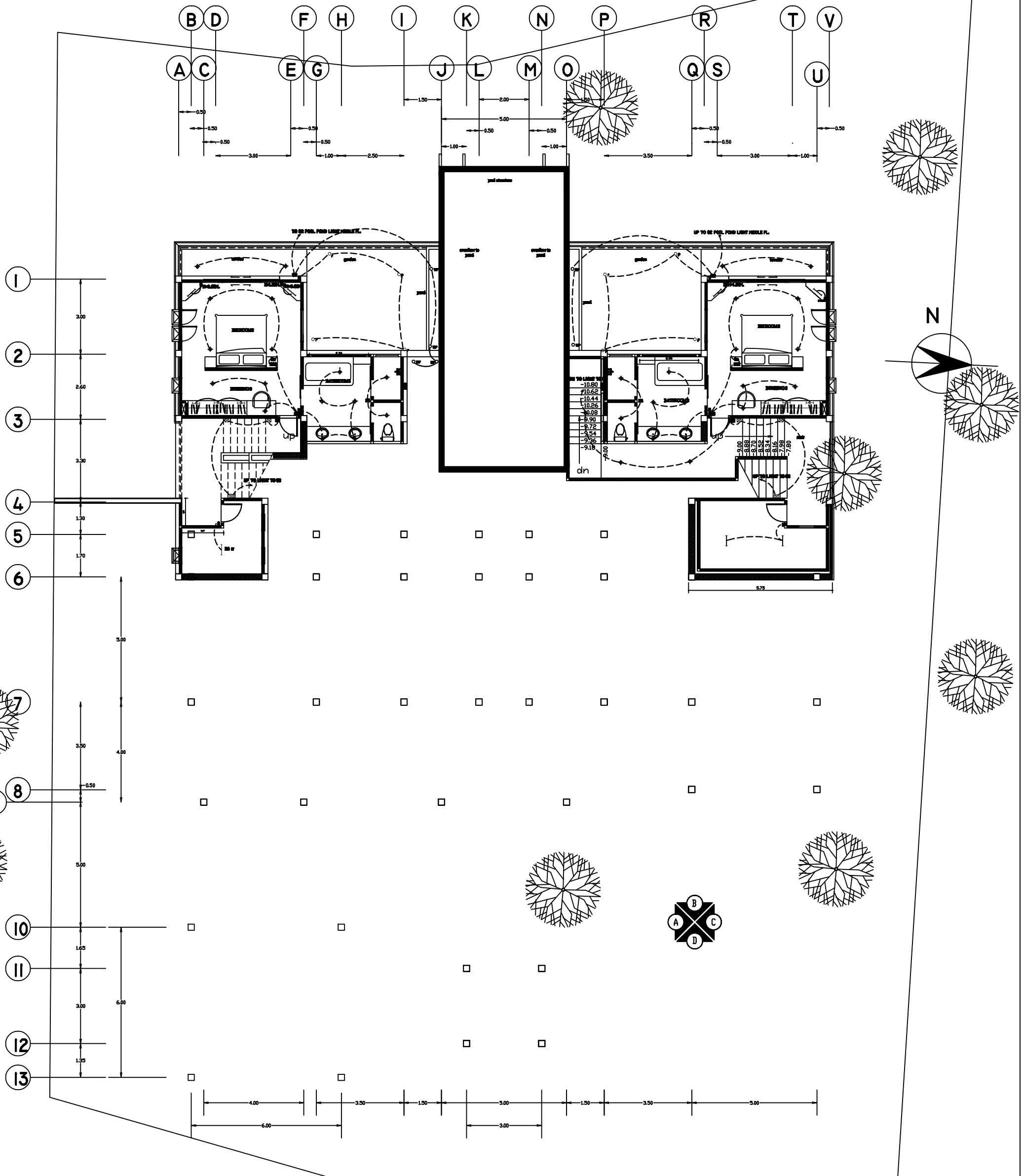
LIGHT ฟังฟืนชั้นล่าง SCALE 1:100
