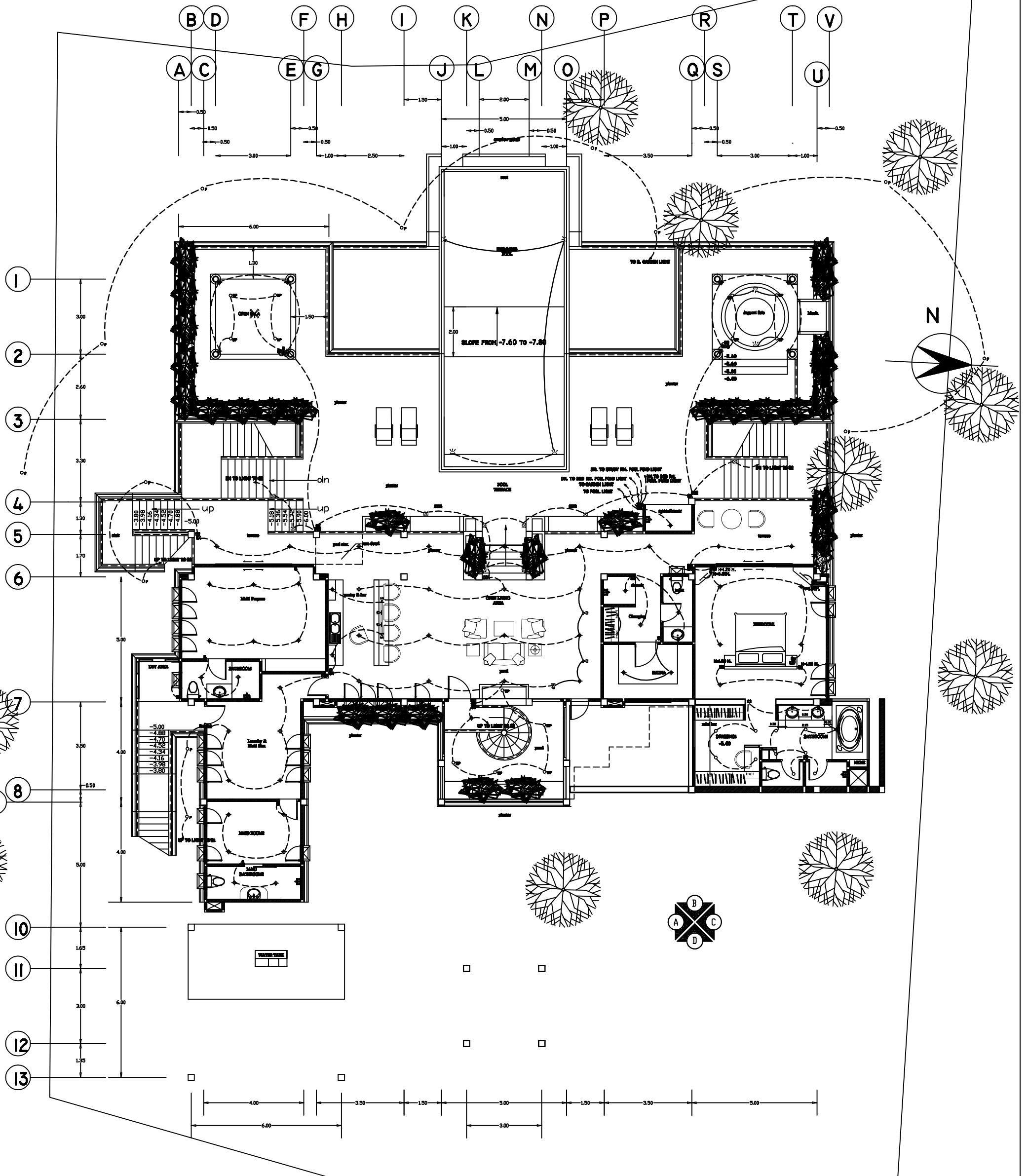
LIGHT ฟังฟืนชั้นกลาง SCALE 1:100
